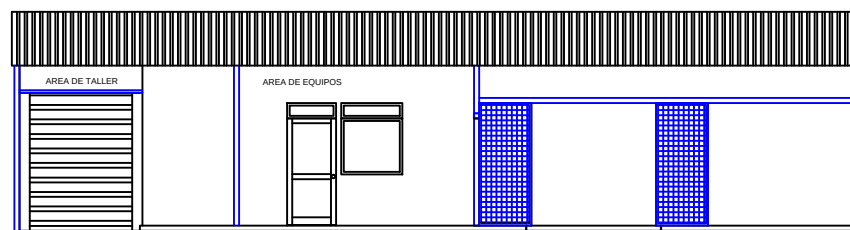
Fachada Frontal Esc 1:50
