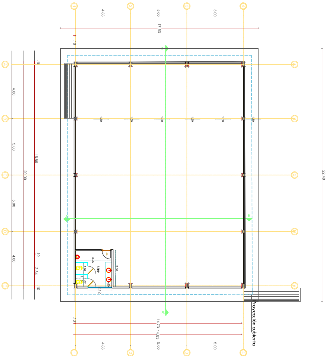
PLANTA BODEGA escala 1:100
